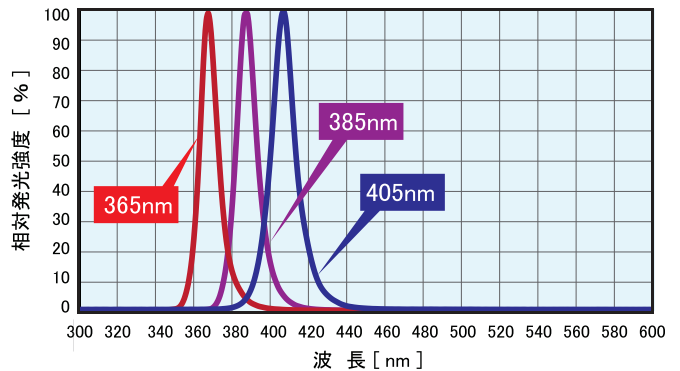
分光特性
